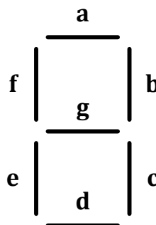
图 2：七段数码管
